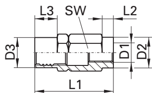
Schraubhülse
