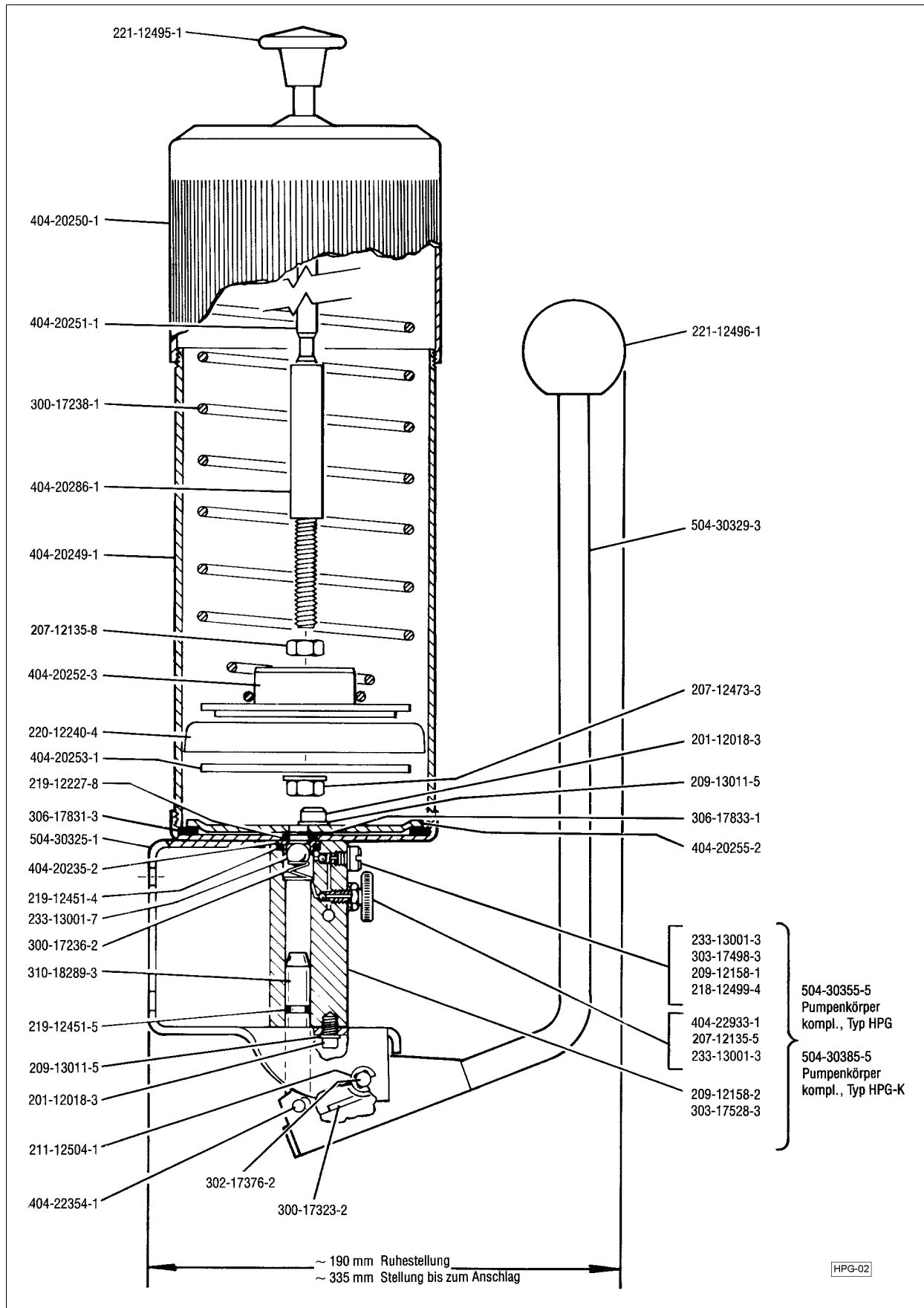
HPG mit 0,4 l Behälter (Seitenansicht)
