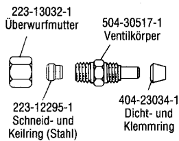
4 mm Rohr – Rückschlagventil
