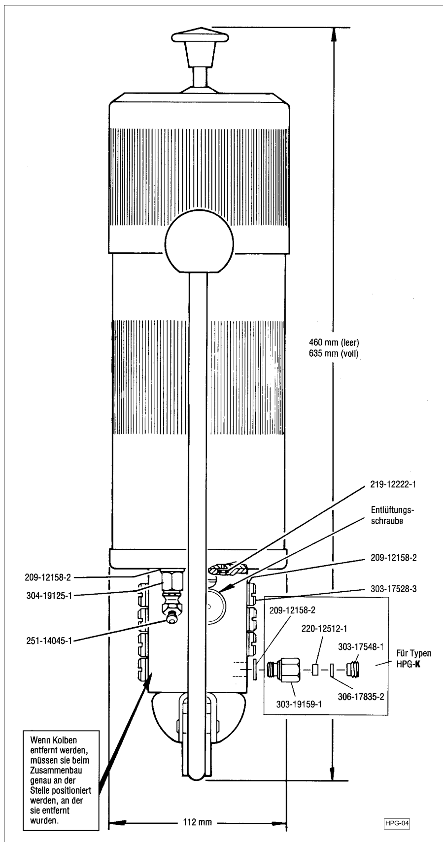
HPG mit 1,5 l Behälter (Vorderansicht)
