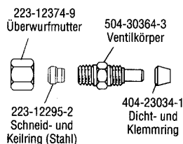
6 mm Rohr – Rückschlagventil
