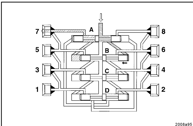
Fig. 11 - Phase 2
