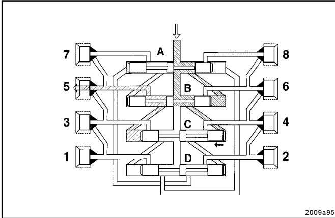
Fig. 12 - Phase 3
