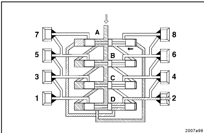
Fig. 10 - Phase 1
