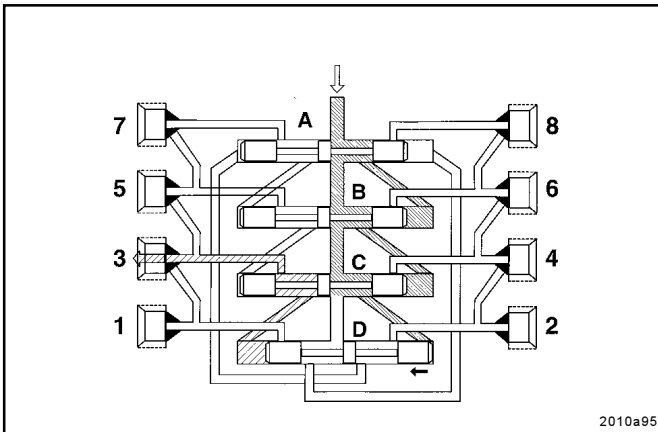
Fig. 13 - Phase 4
