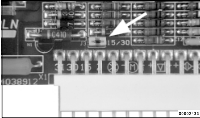
Abb. 6 - Jumper 15/30 aufgesteckt
