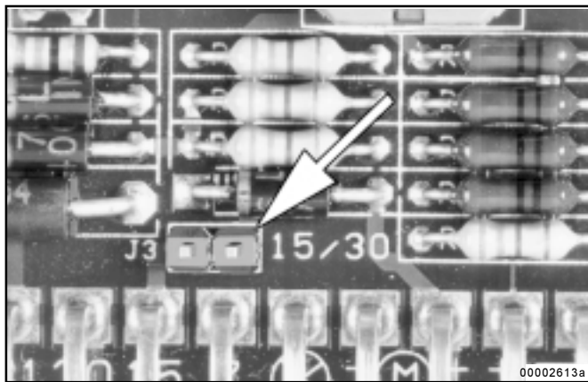
Abb. 7 - Jumper 15/30 entfernt
