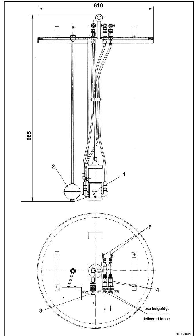
Fig. 2.4.2: Pompe pneumatique sur fût SAF2
