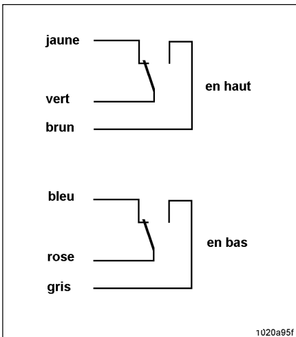
Fig. 2.5.1: Code des couleurs des câbles de connexion
