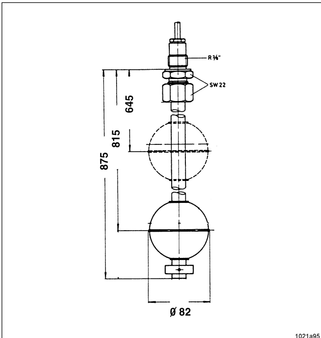
Fig. 2.5.2: Schéma coté
