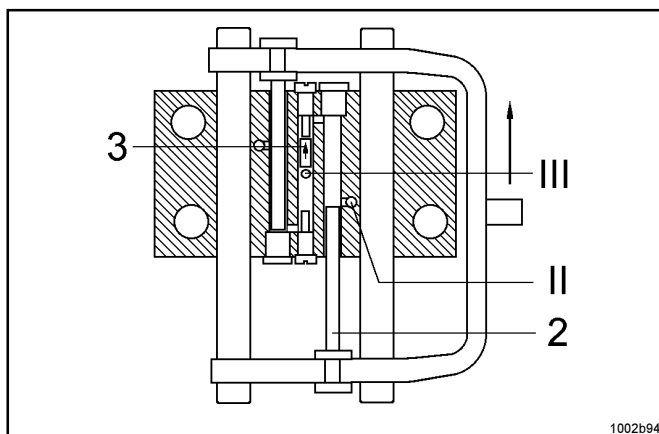
Abb. 2.6.3: untere Endstellung
