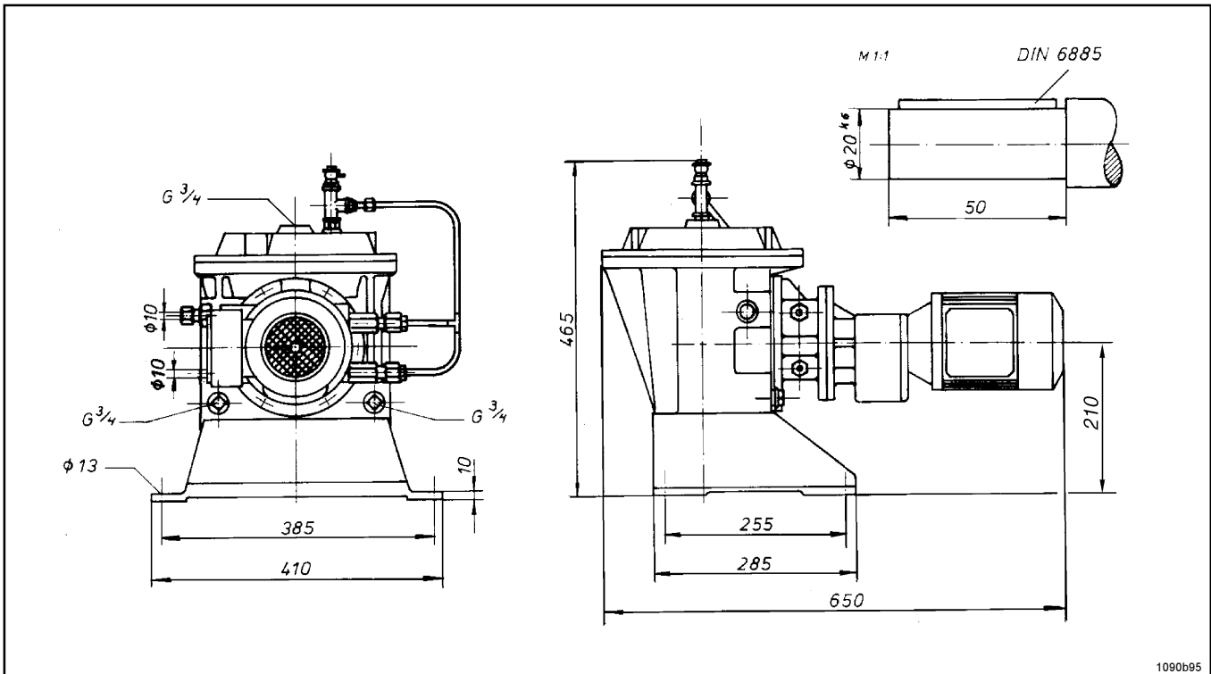
Abb. 6.2.1: Maßzeichnung ZPU09A
