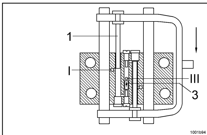
Abb. 2.6.1: obere Endstellung
