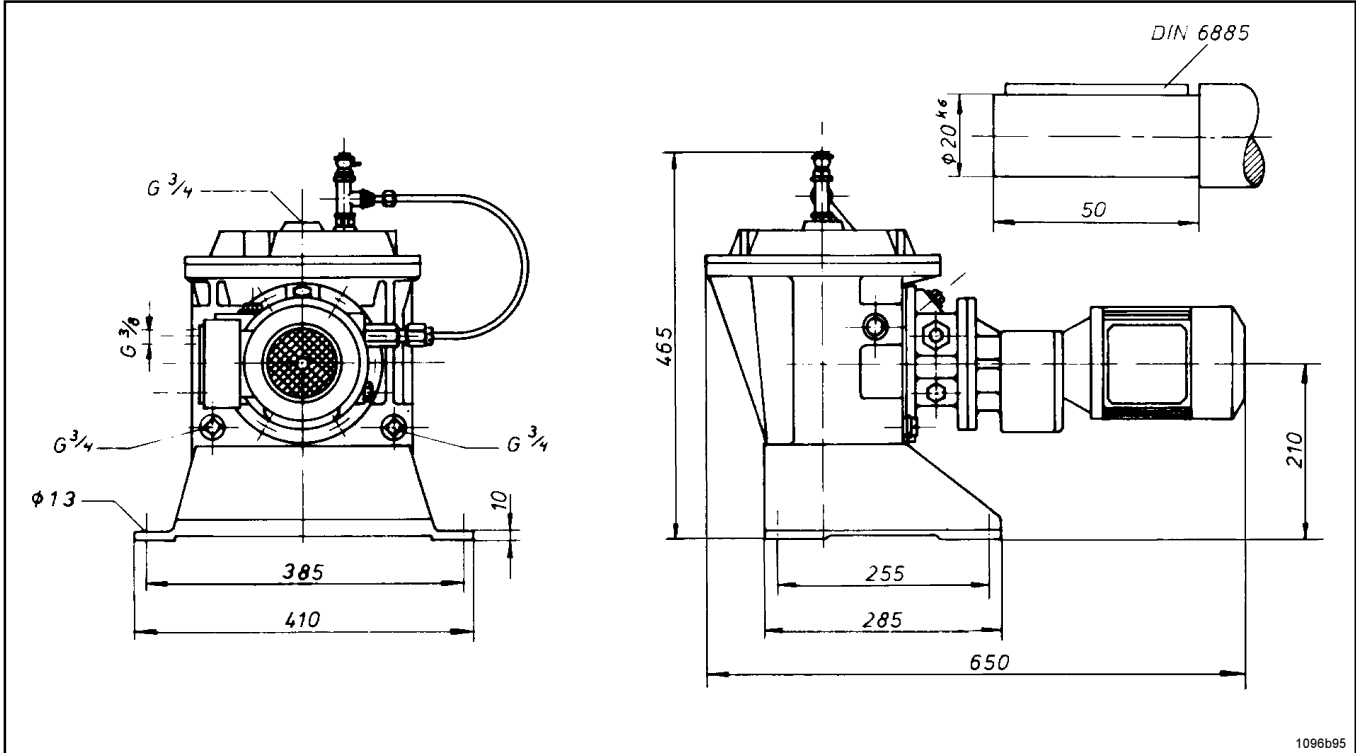
Abb. 6.2.1: Maßzeichnung ZPU09
