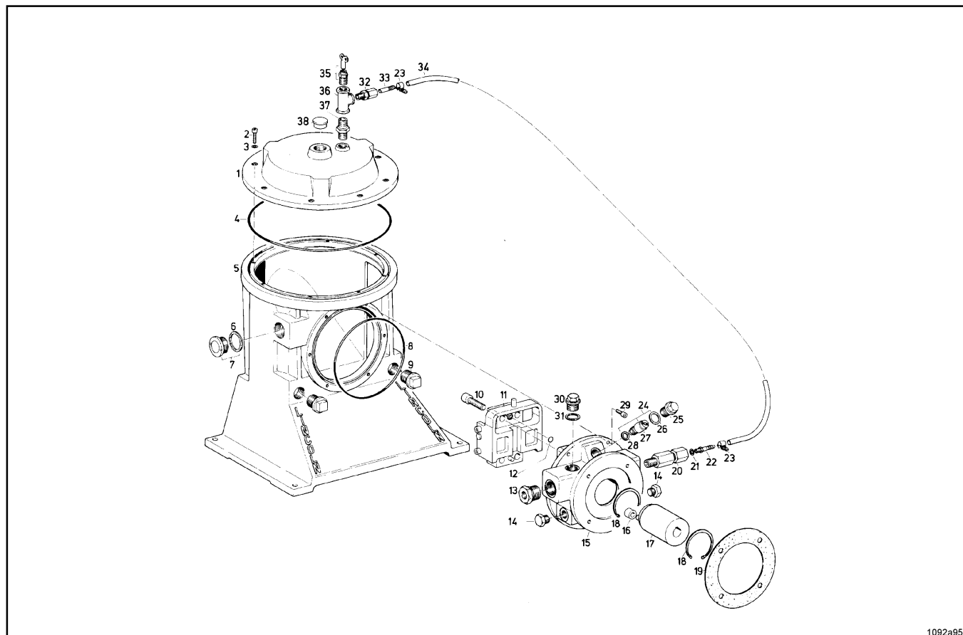
Abb 5.1.1: Hochdruck Zentralschmierpumpe ZPU 09
