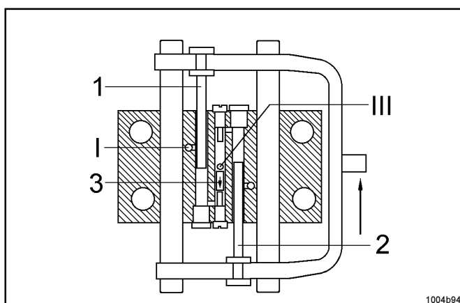
Abb. 2.6.4: Arbeitshub aufwärts
