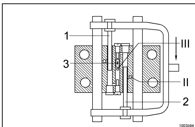
Abb. 2.6.2: Arbeitshub abwärts
