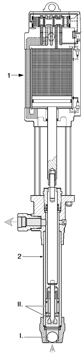
I Soupape de pied à bille II Piston
