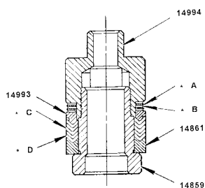
Kolben-Garnitur Nr. 84112 (Pos. 22-29)
