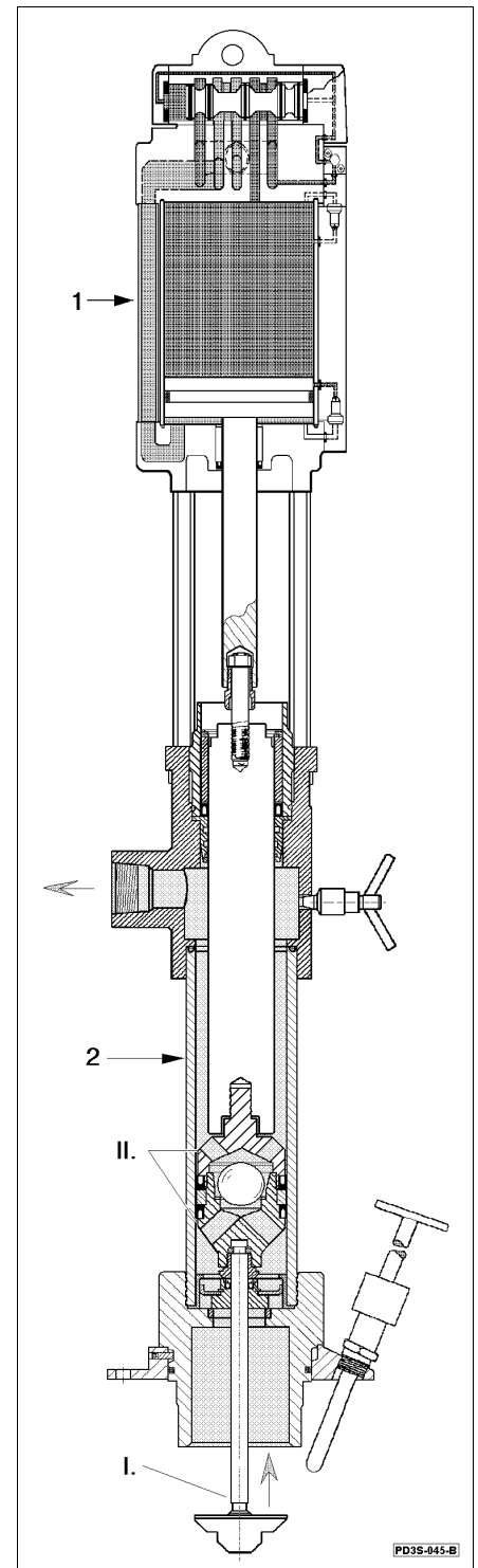
1 Luftmotor 2 Pumpenrohr I Schöpfkolben II Kolben
