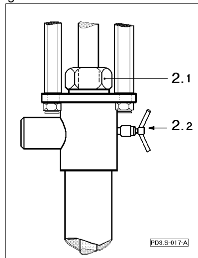
2.1 Schmierbüchse 2.2 Entlüftungsventil
