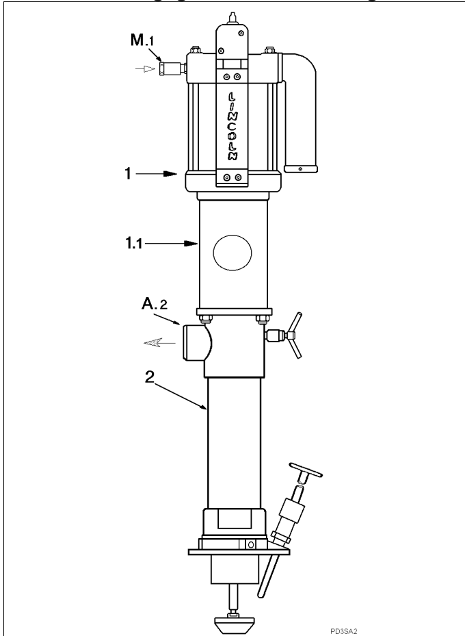
Pile Driver III Pumpe mit Power Master III Luftmotor
