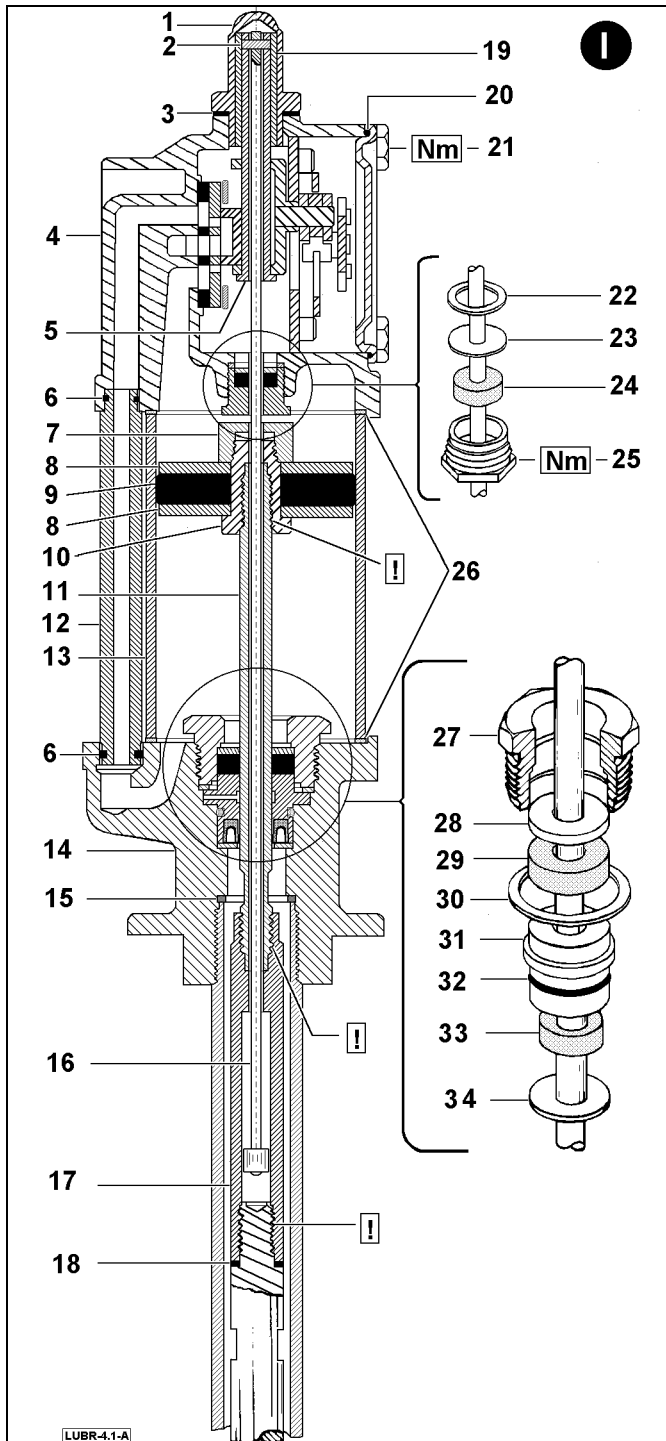
Ersatzteilzeichnung 1 von 3
