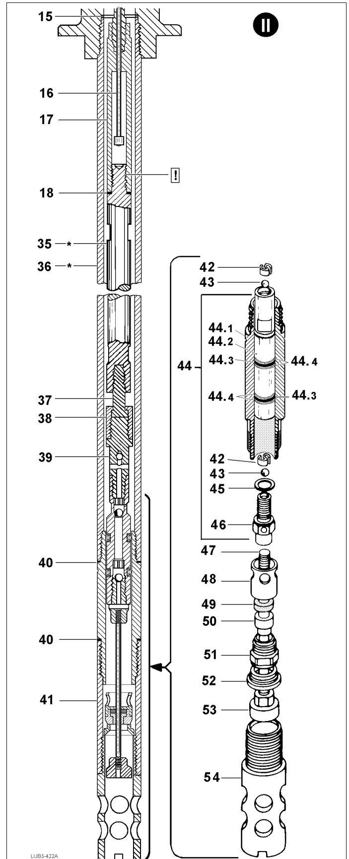
Ersatzteilzeichnung 2 von 3
