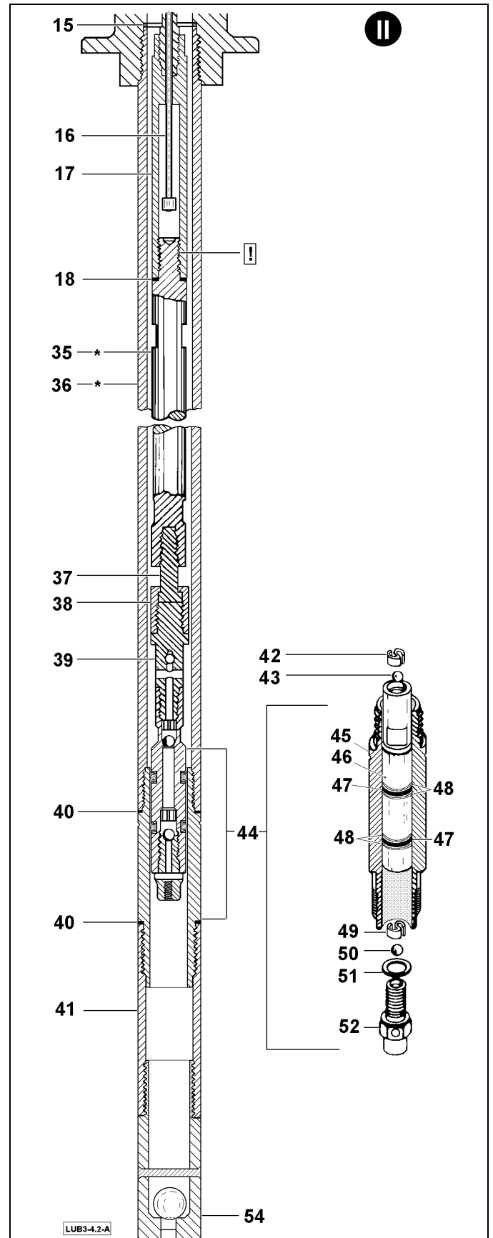
Ersatzteilzeichnung 2 von 3
