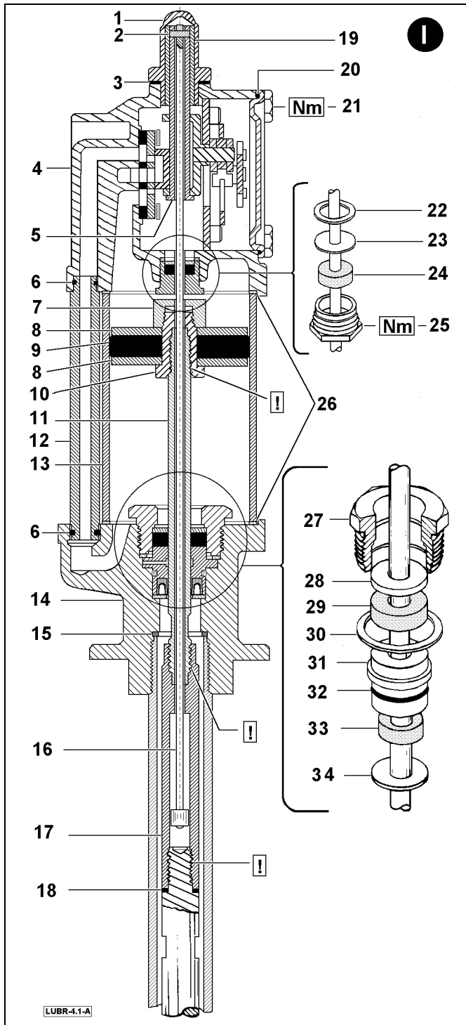
Ersatzteilzeichnung 1 von 3
