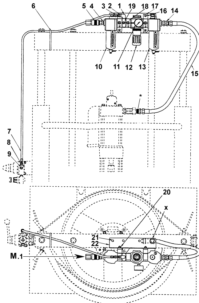
M.1 Luftanschluß (Schnellkupplung) 1/2" NPTF innen
