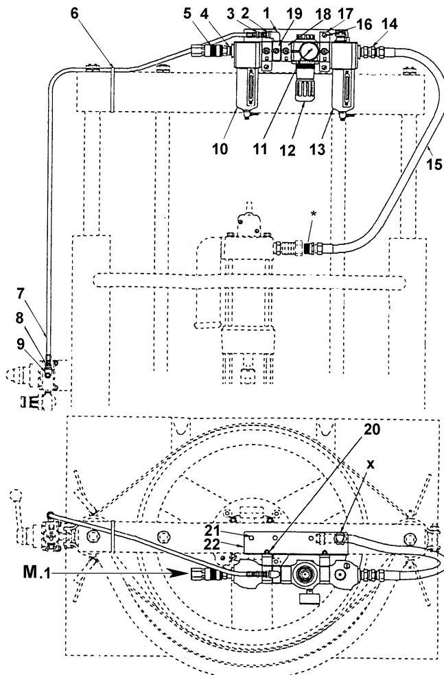
M.1 Luftanschluß (Schnellkupplung) 1/2" NPTF innen
