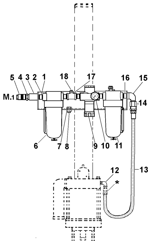
M.1 Luftanschluß (Schnellkupplung) 3/4" NPTF innen
