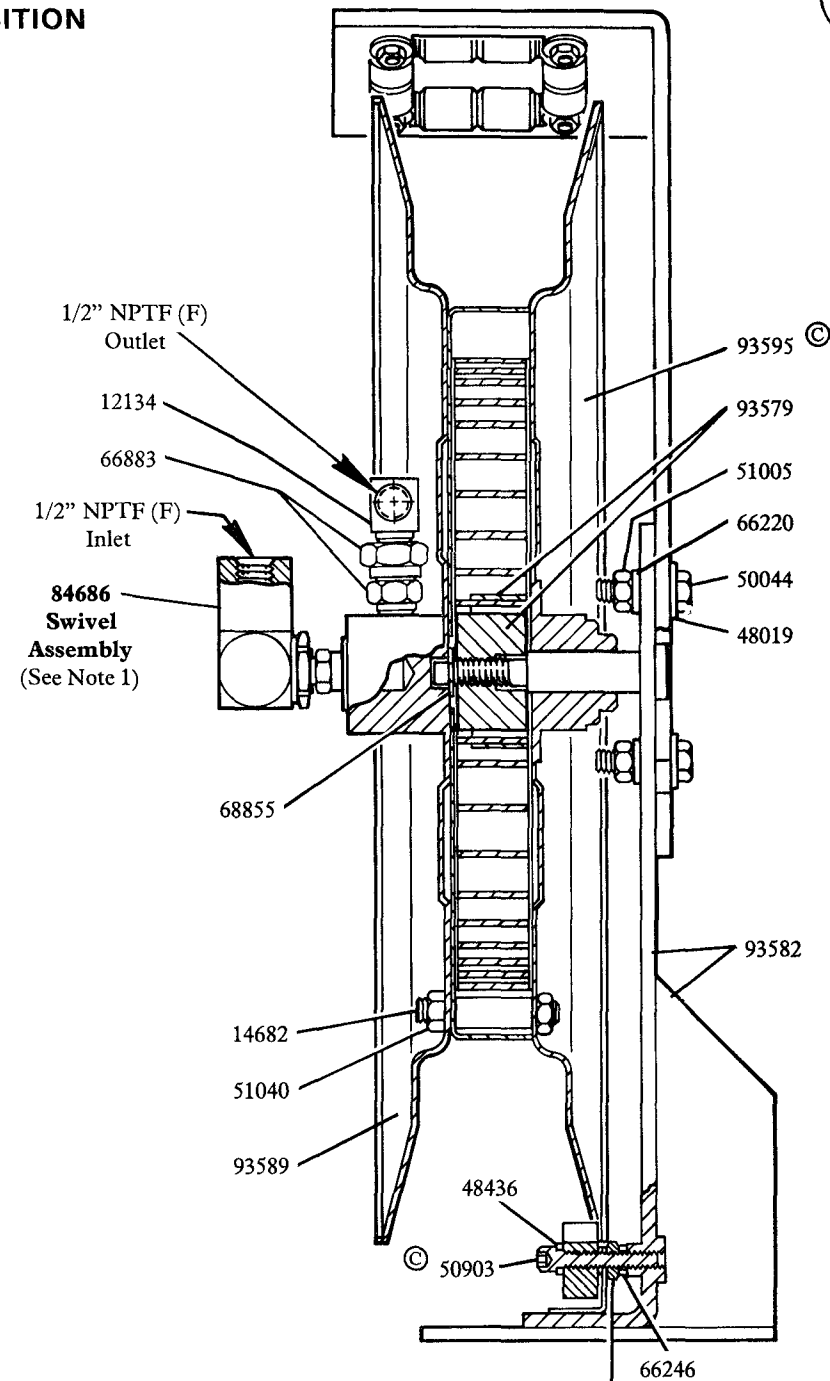
SECTION A-A
